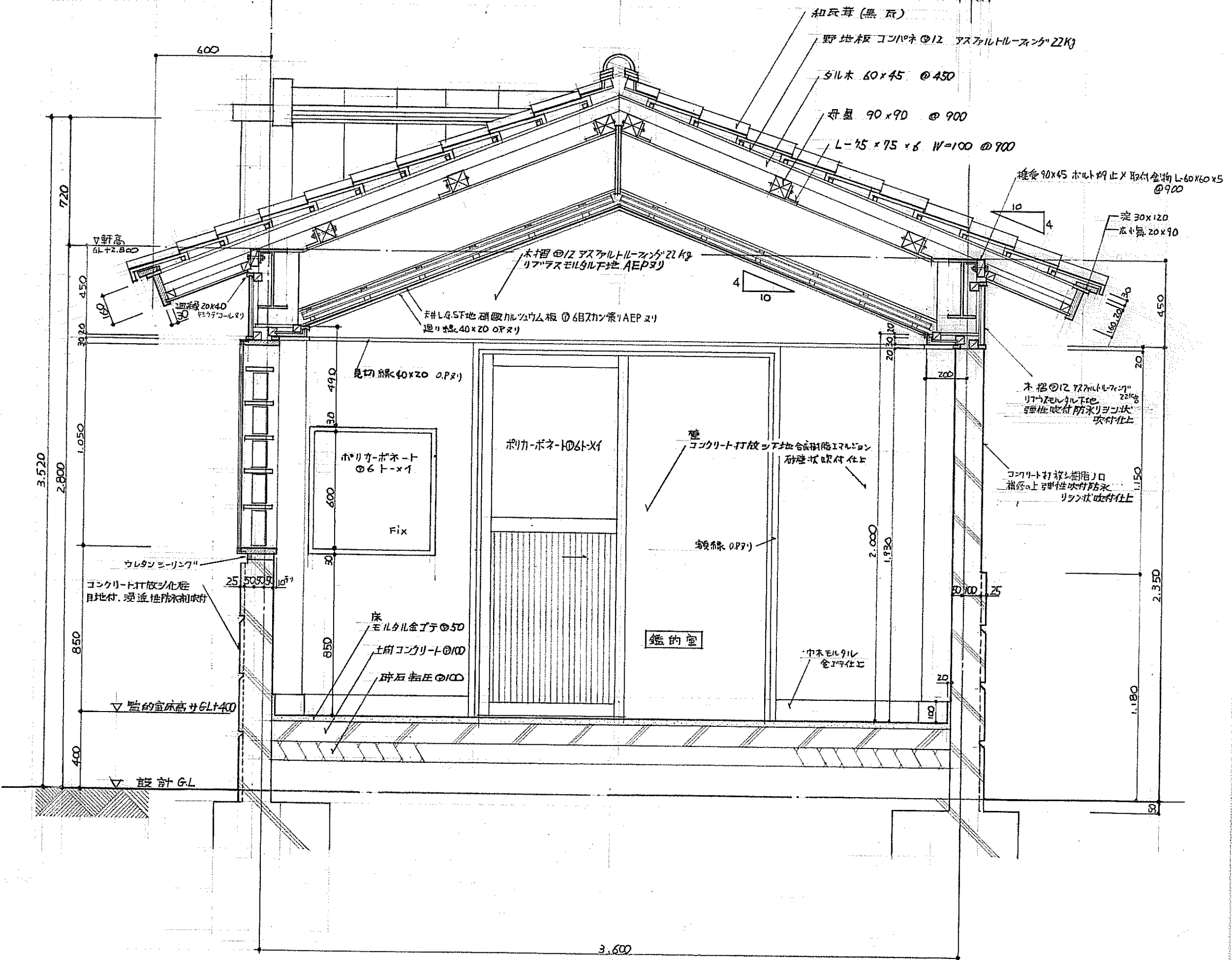
的場棟矩計図 1/20
