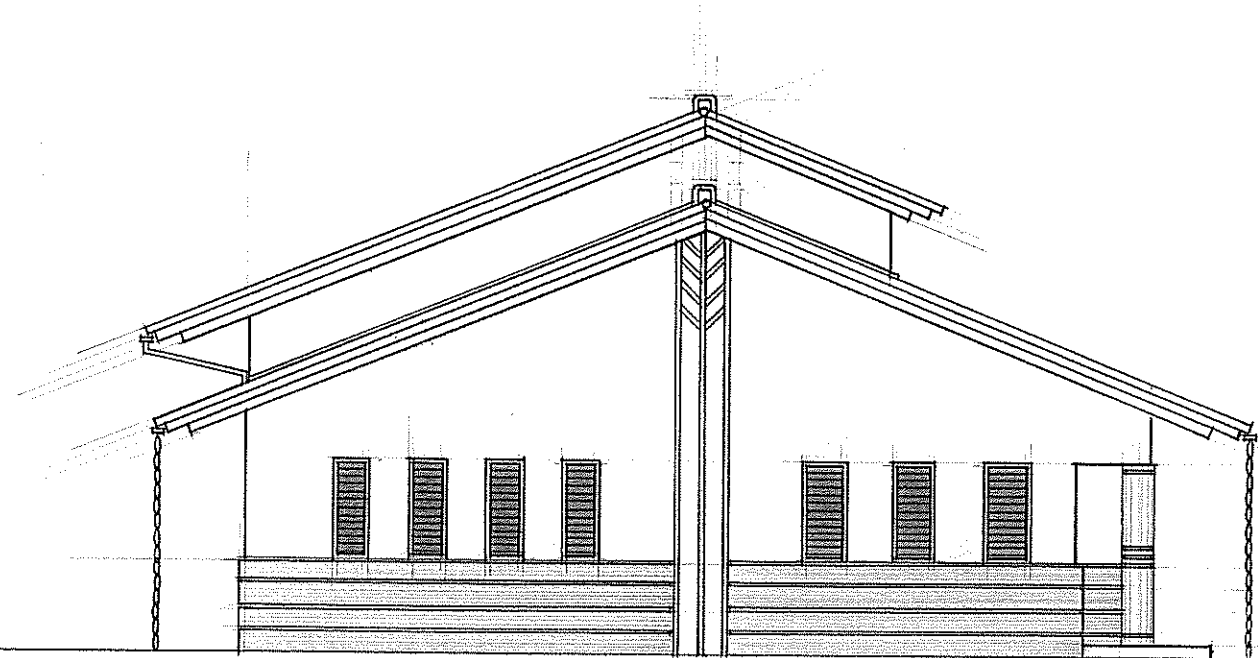
東立面図
