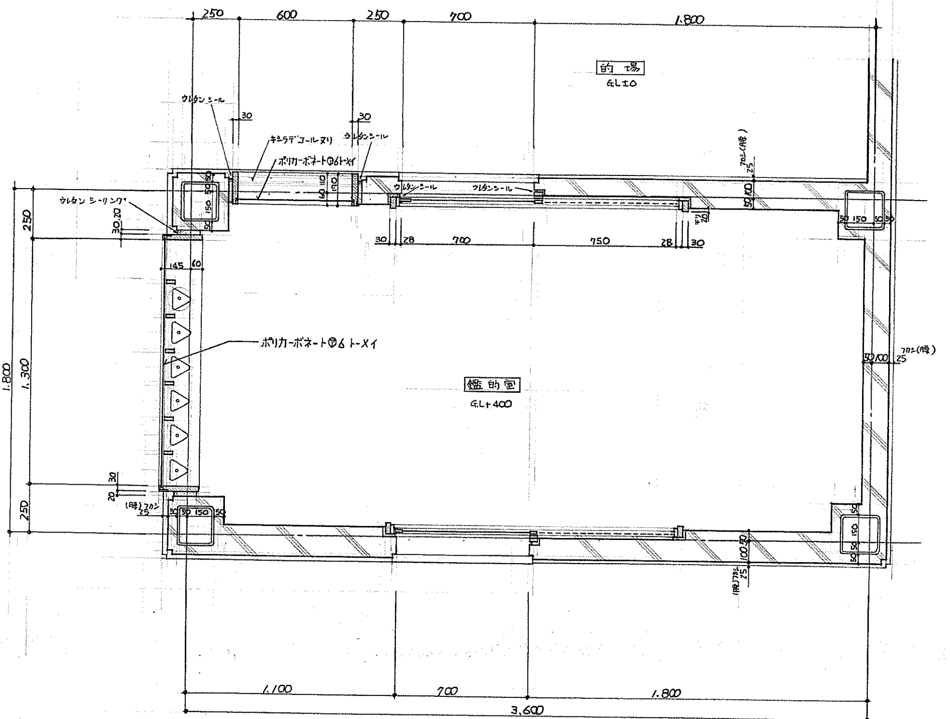
的場棟平面詳細図 1/20
