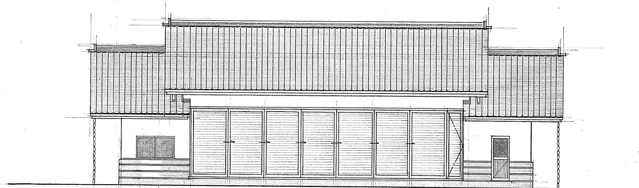
西立面図
