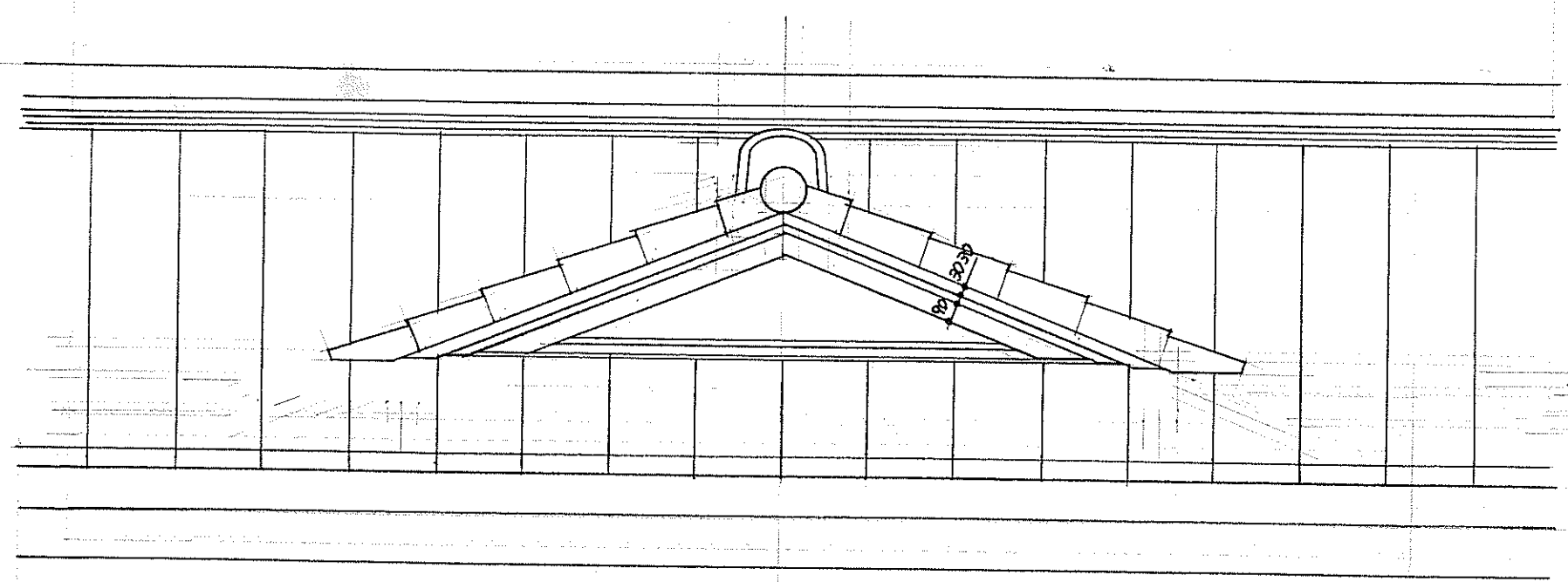
立面图 1/20
